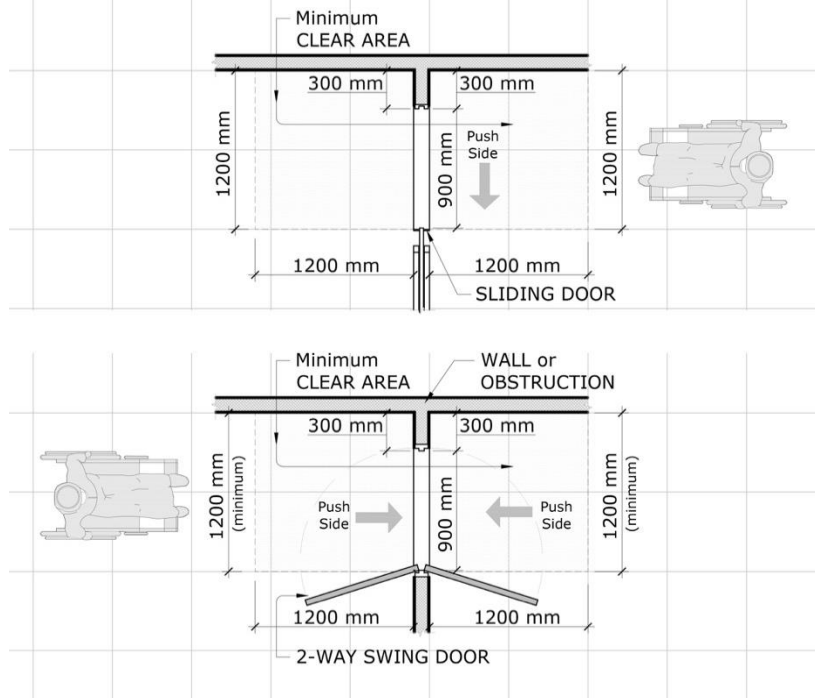
Figure 29. Door clear spaces
